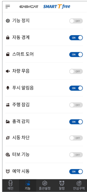
<기능 화면>
