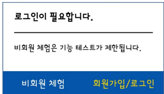
[비회원체험/회원가입/로그인 팝업창]
