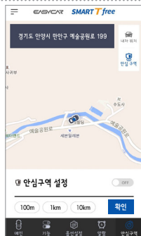
<안심구역 화면>
