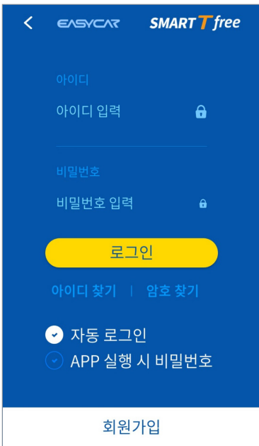
<회원가입/로그인 화면>
